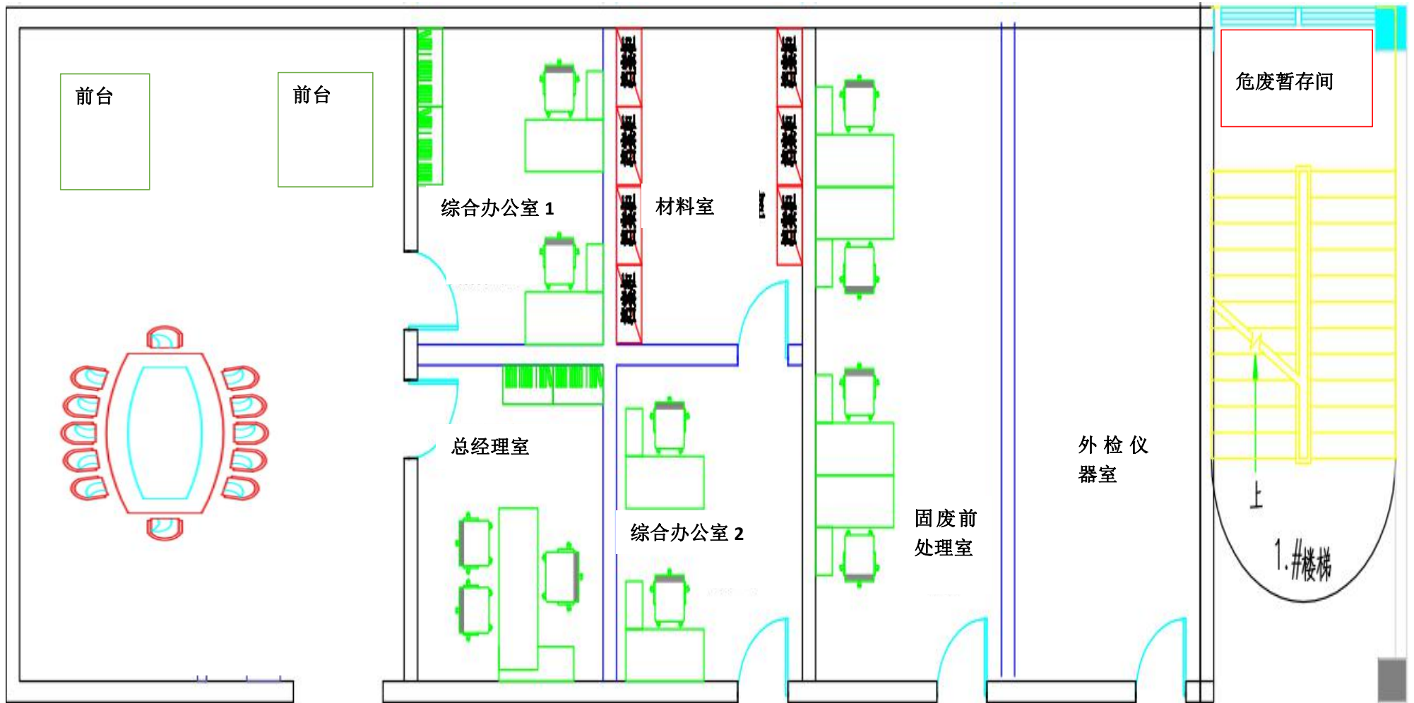
附图 4-1 一层布置图
