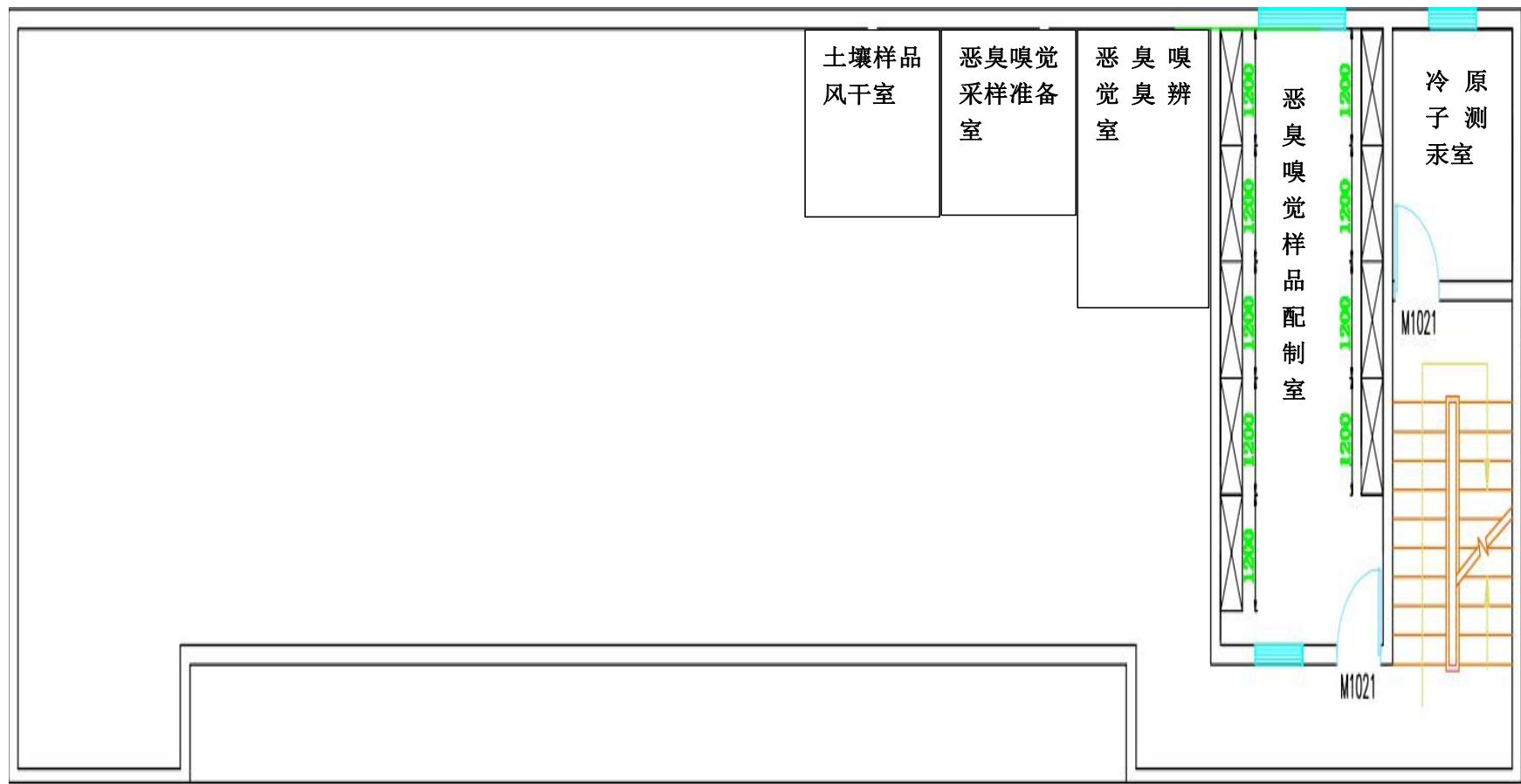
附图 4-4 四层实验室布置图
