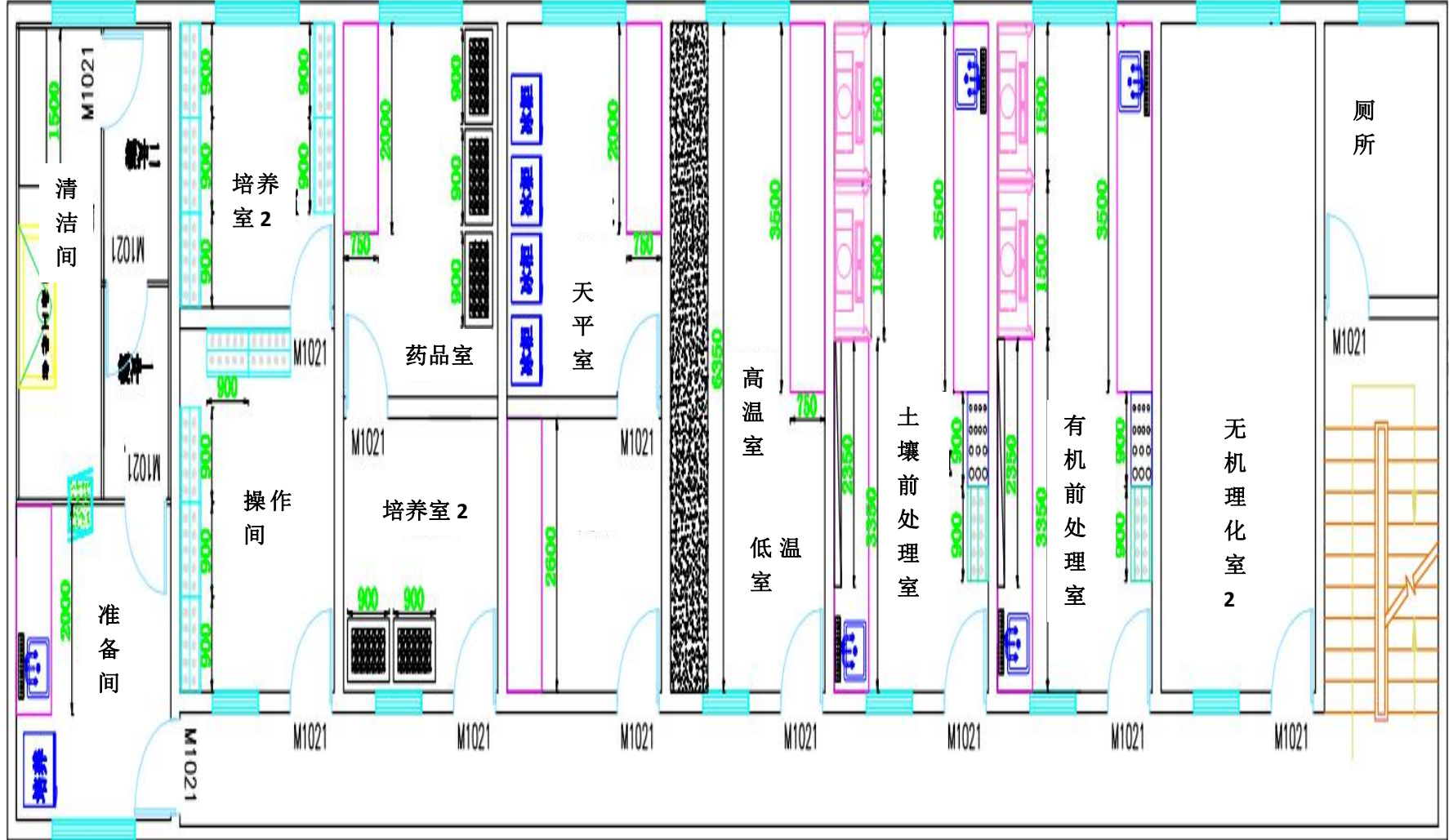
附图 4-3 三层实验室家具布置图
